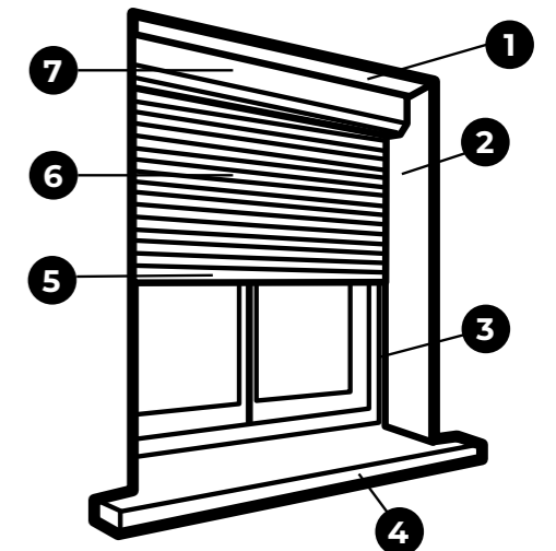
1 Linteau 2 Tableau 3 Coulisse 4 Appui 5 Lame finale 6 Tablier 7 Coffre
